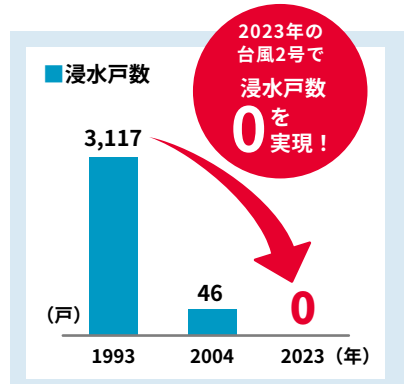
図1：神田川・環状七号線地下調節池の整備効果
